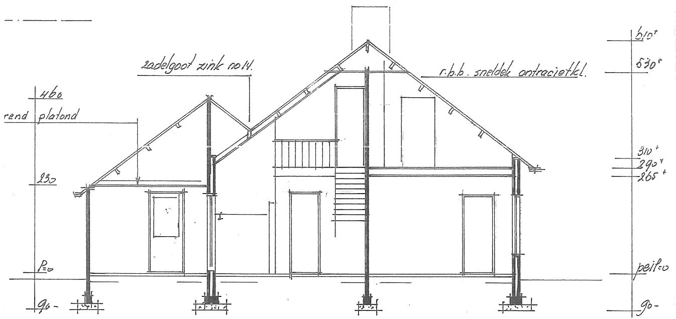
DOORSNËDE A - B
