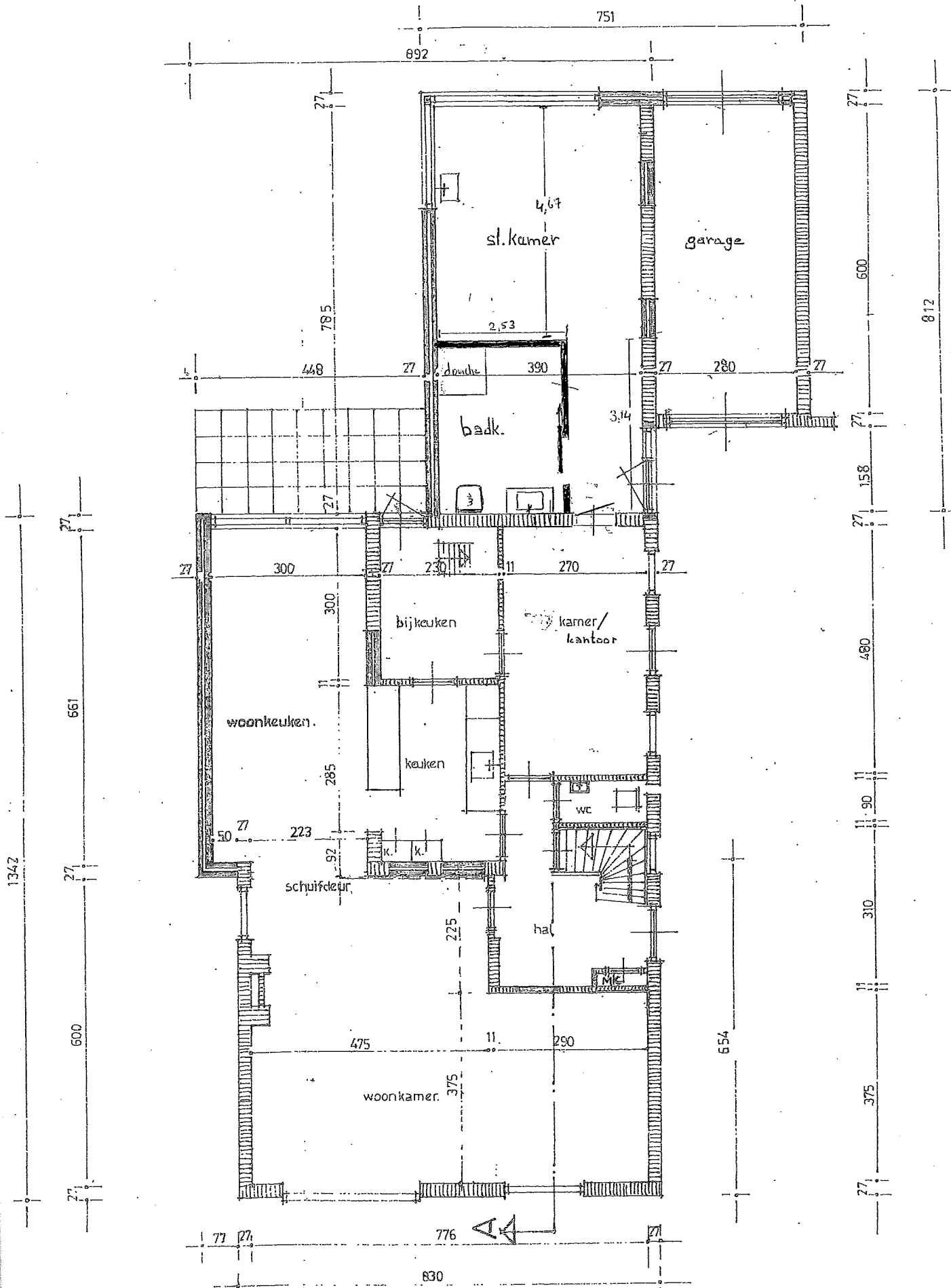
plattegrond BG
