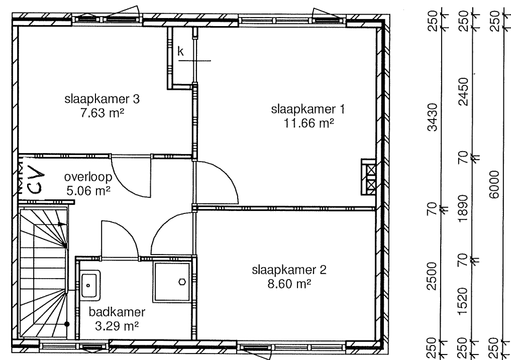
110 3350 90 3440 250 110 1116 70 2164 90 3440 250 110 6880 250 eerste verdieping
